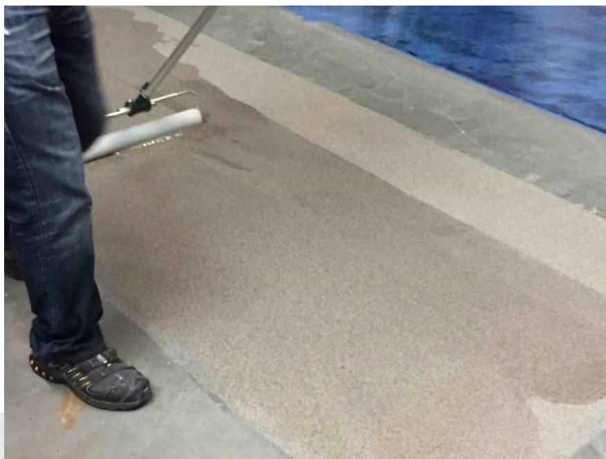
Foto: Aanbrengen primer.
